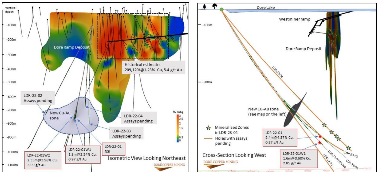
Abbildung 1. Isometrische Ansicht und Querschnitt der Lagerstätte Doré Ramp mit der Lage der neuen Kupfer-Gold-Mineralisierungszone (LDR-22-01W2 korrigiert)
